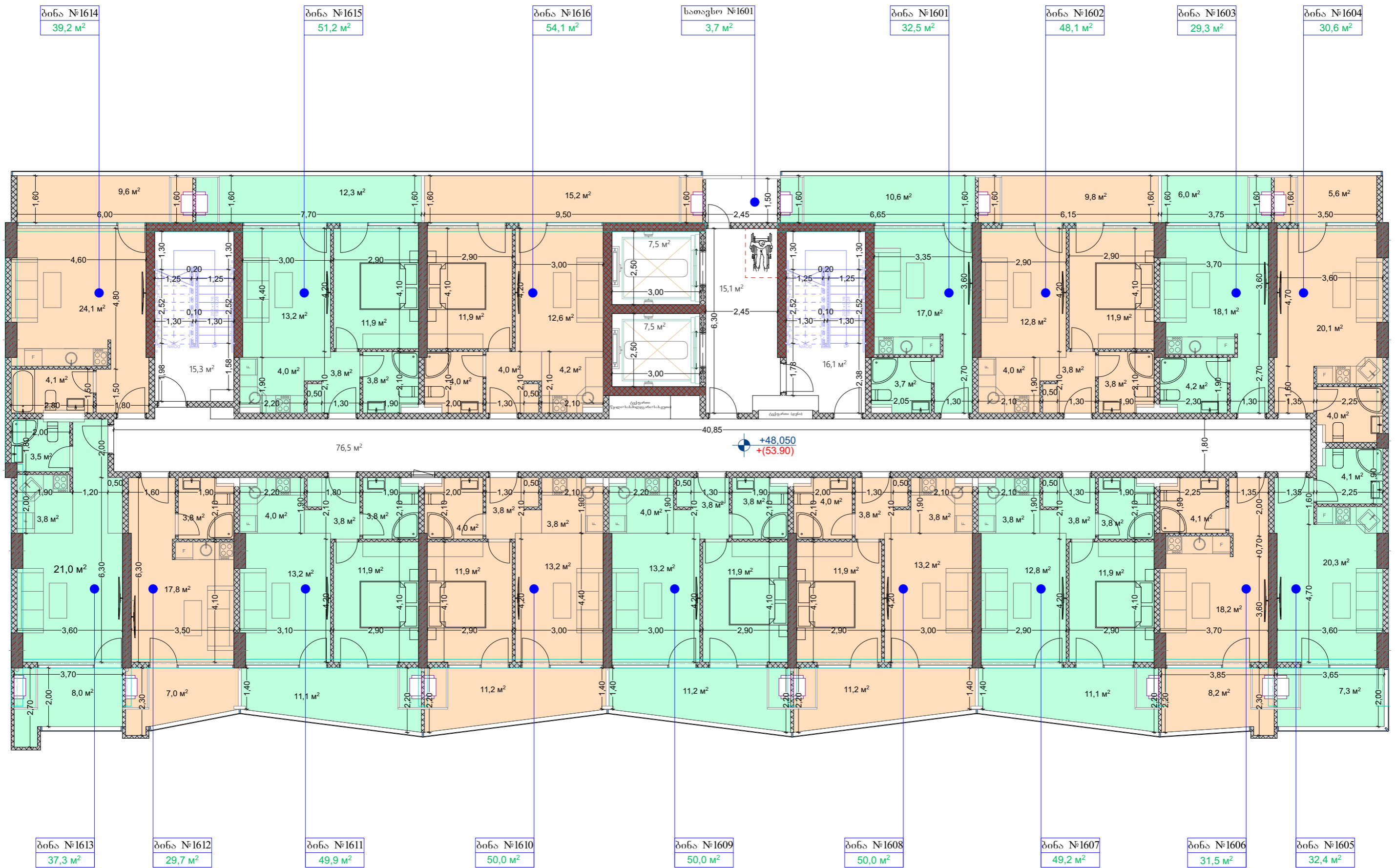
მეთექვსმეტე სართული
